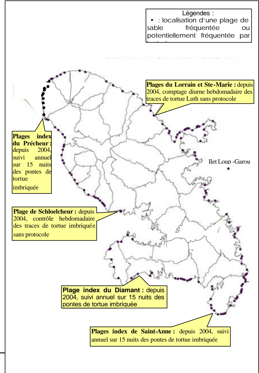
Carte 4 : Localisation des plages de Martinique faisant l'objet d'un suivi des populations de tortues marines
