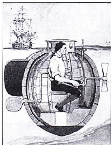
Dessin en coupe du 'Turtle'
